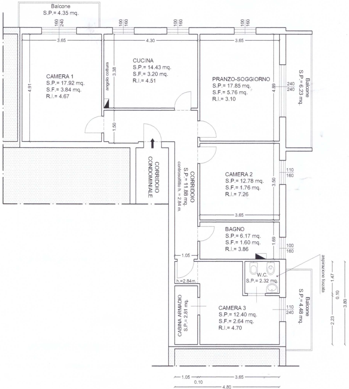
PIANTA PIANO QUINTO - H = 3.00 ml
